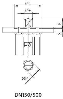
DN150/500
