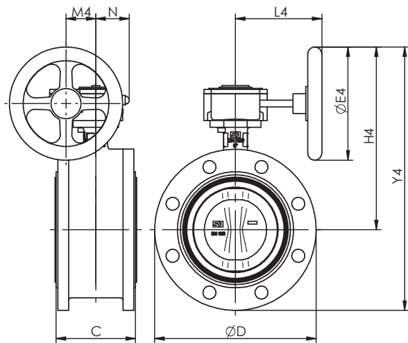
MDV - převod s ručním kolem MDV - gearbox with handwheel
