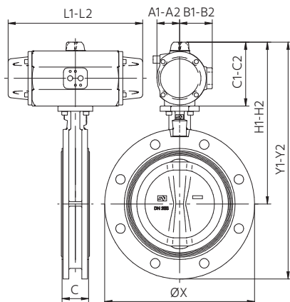
MND - 2-činný pneumatický pohon / double acting pneumatic actuator
