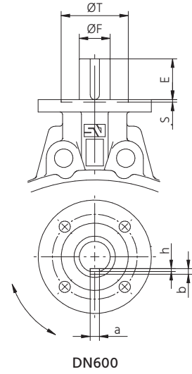
DN600
