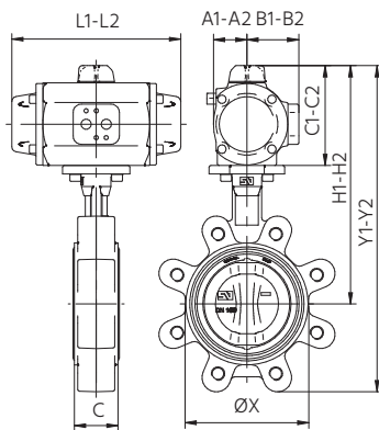
MND - 2-činný pneumatický pohon / double acting pneumatic actuator MNS - 1-činný pneumatický pohon / spring return pneumatic actuator
