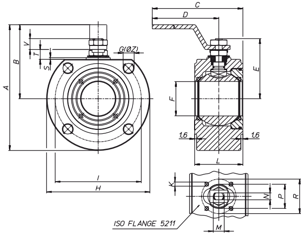
Fig. 3 DN15–DN100 ..... JADE type
