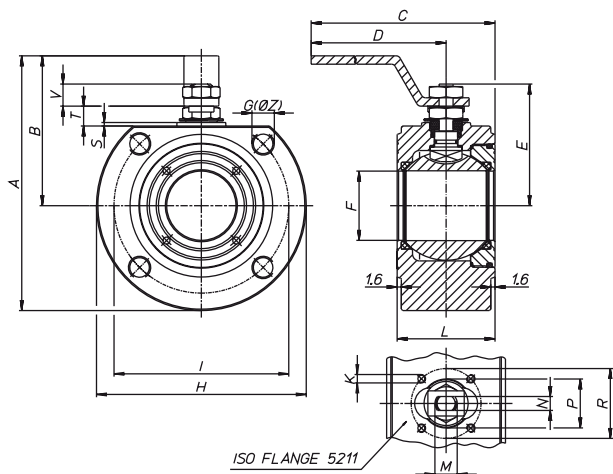
Fig. 2 DN 15–DN 100
